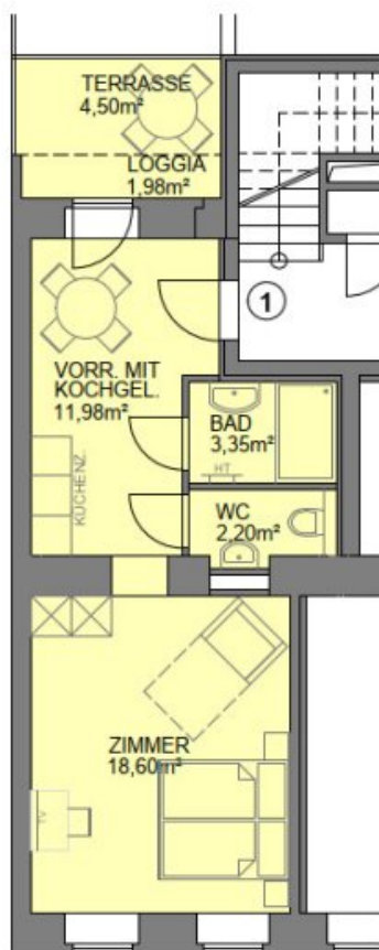
GRUNDRISS M1:100
