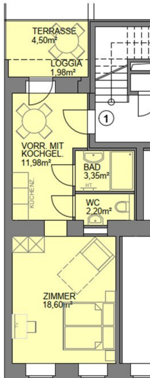
GRUNDRISS M1:100
