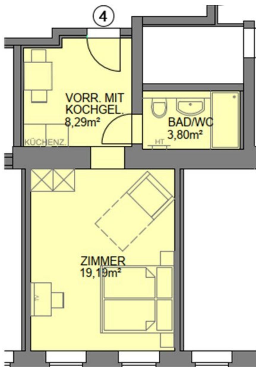
GRUNDRISS M1:100
