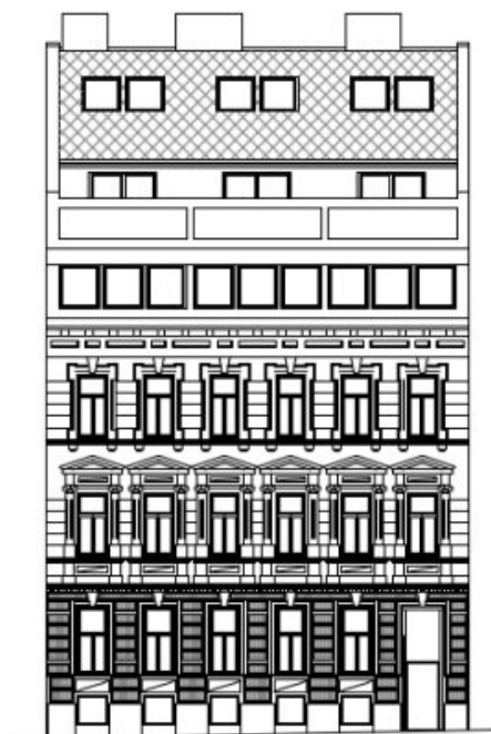
STRASSENFASADE M1:200
