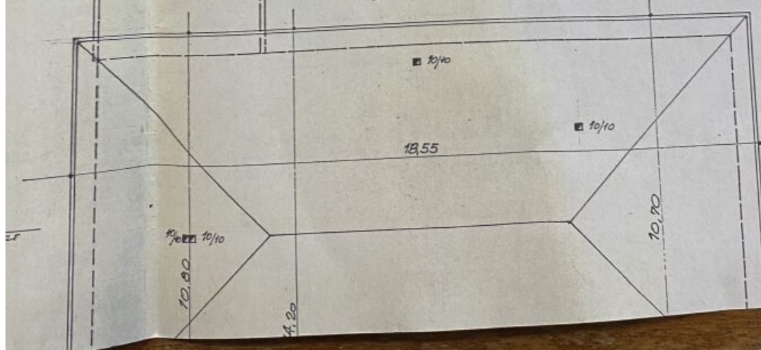
GRUNDRISS OBERGESCHOSS.
