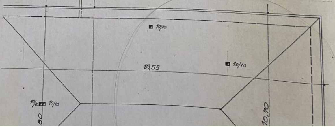
GRUNDEISS OBERGESCHOSS.
