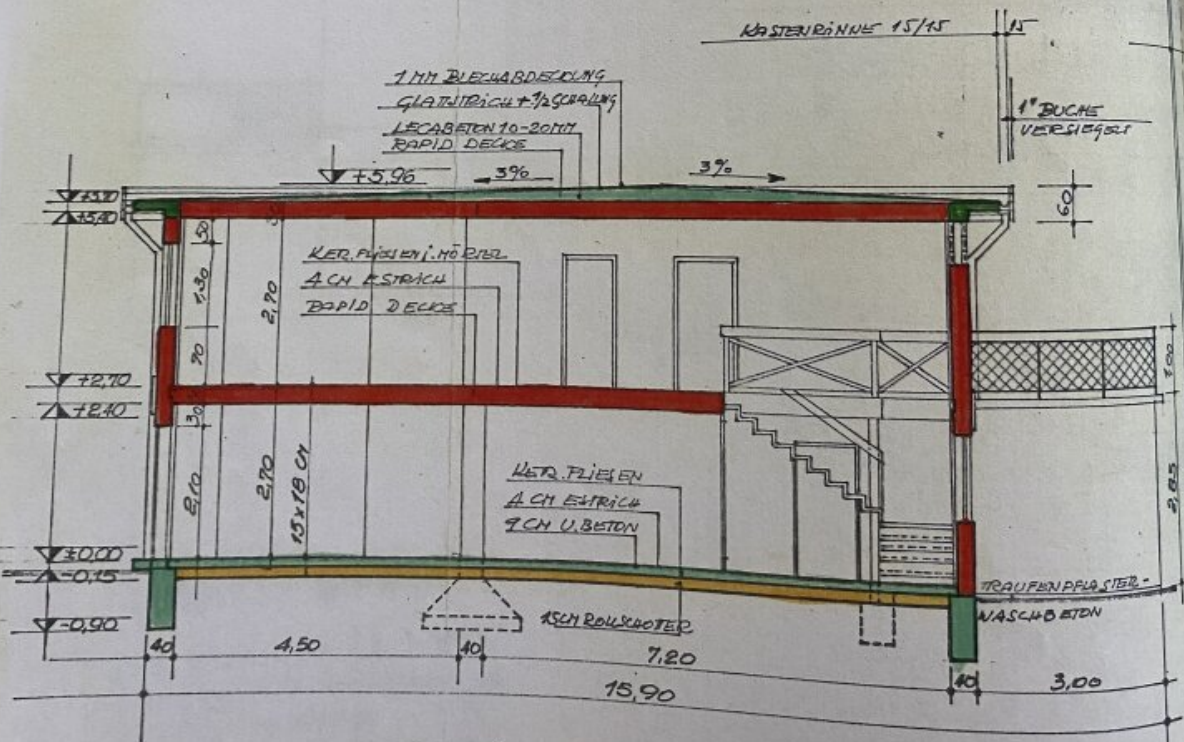
SCHNITT A-A:
