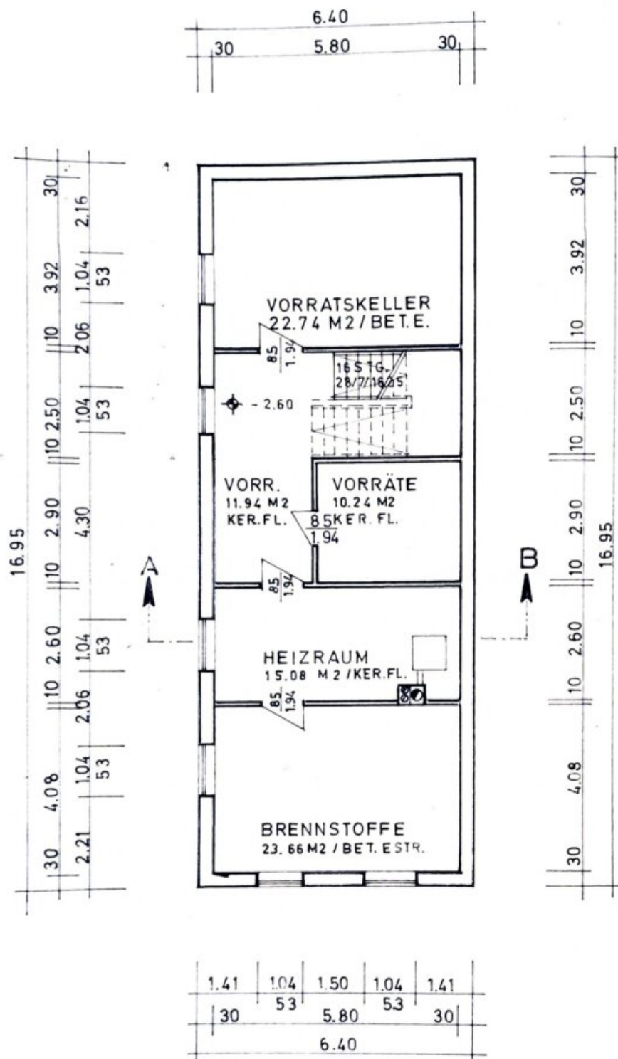
KELLERGECHOSS
