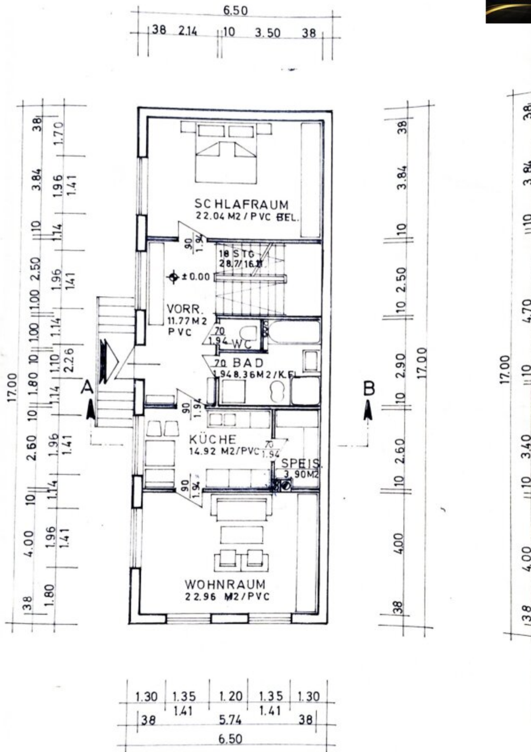
ERDGESCHOSS
