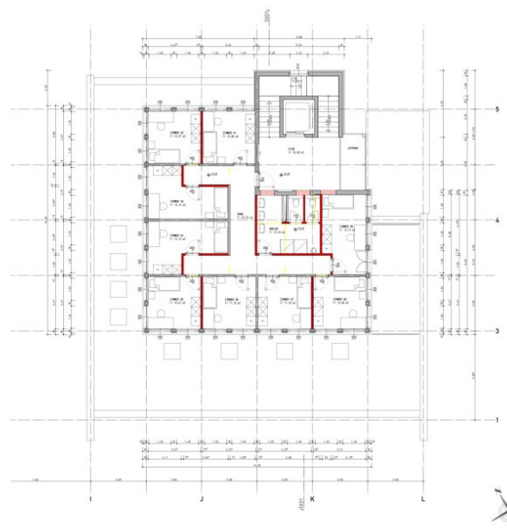
4. OBERGESCHOSS
