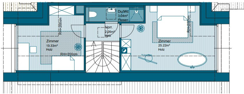
Dachgeschoss
