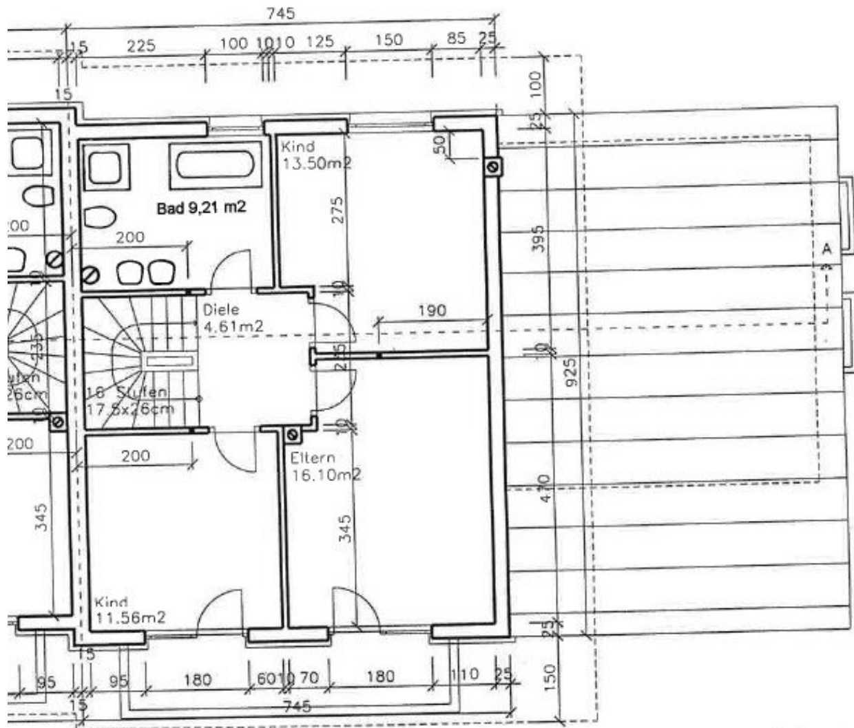
OBERGESCHOSS 1:100
