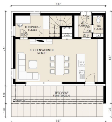
ERDGESCHOSS
