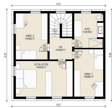
OBERGESCHOSS
