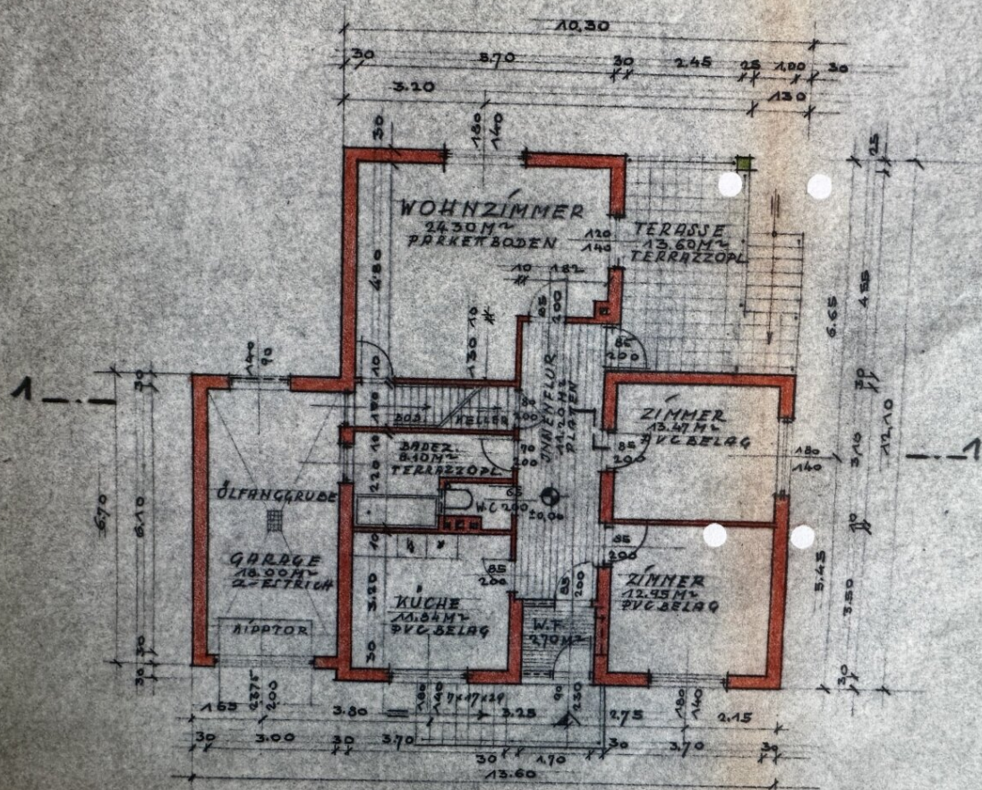
ERDGESCHOSS
