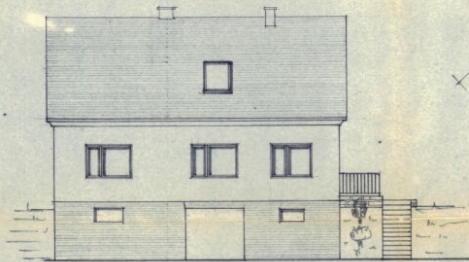
NORDOSTANSICHT
