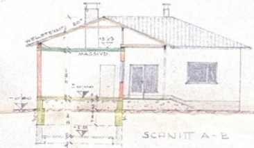
SCHNITT A-B
