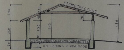
SCHNITT A-B
