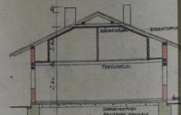
SCHNITT A-B
