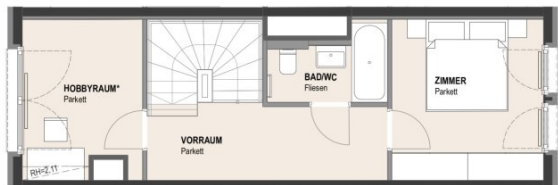
ERDGESCHOSS
