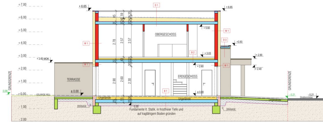
SNITT B-B
