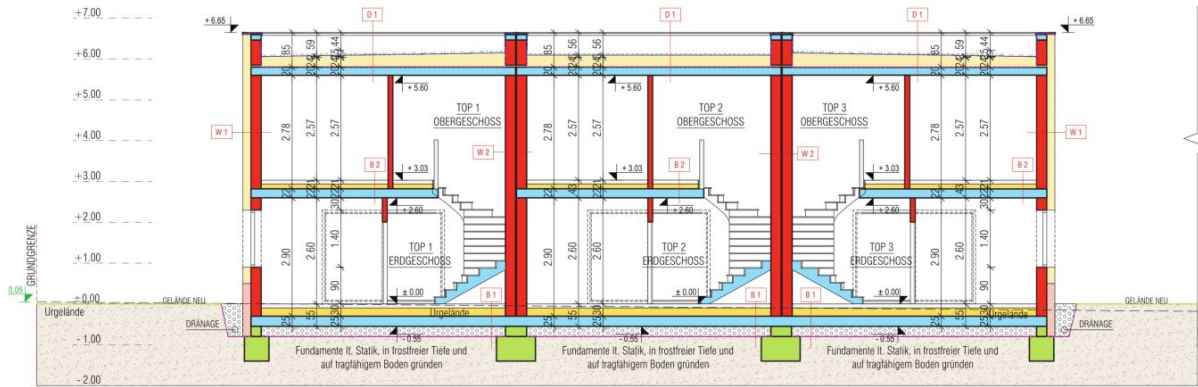
SNITT A-A
