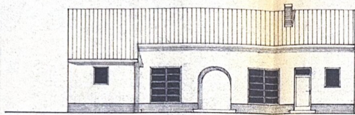
SÜD-ANSICHT
