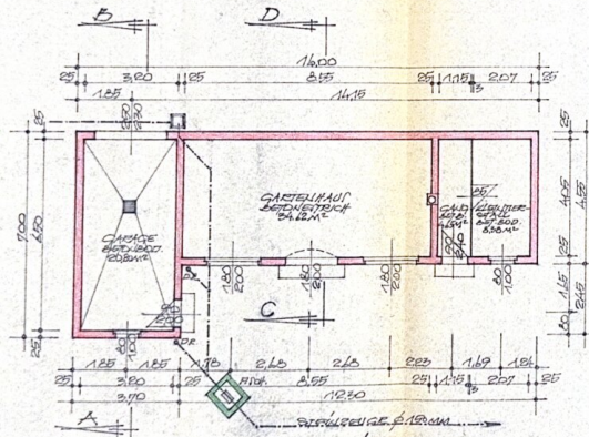
GRUNDRIß
