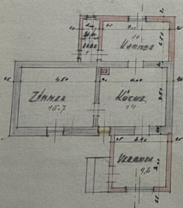
EGGESCHOSSE
