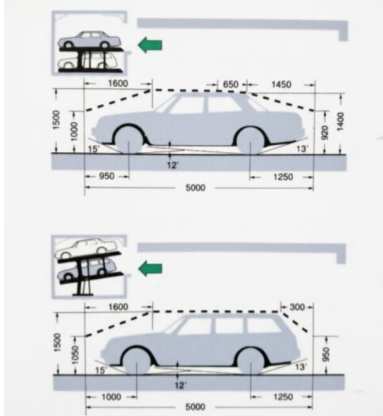
Zugelassene PKW-Maße für die Standardanlage
