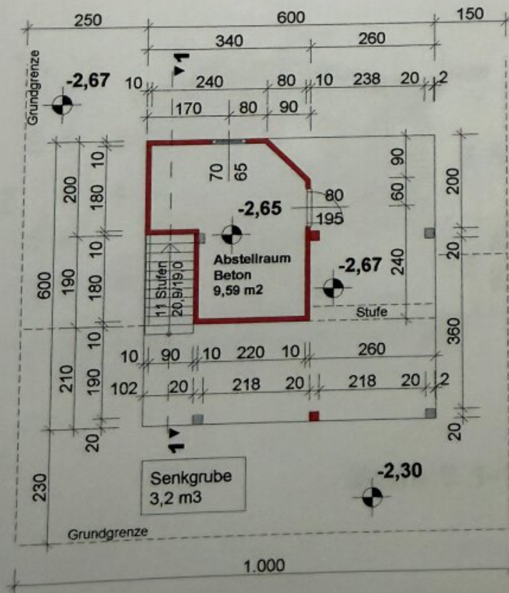
Erdgeschoß
