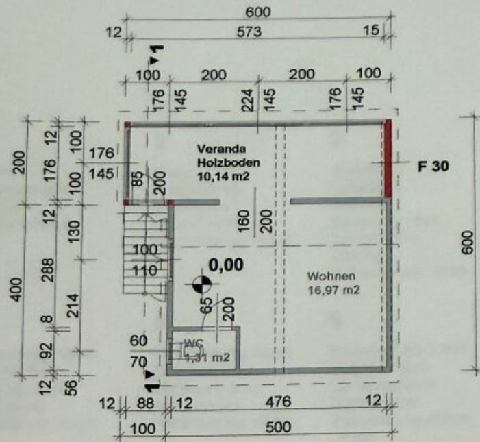
Obergeschoß
