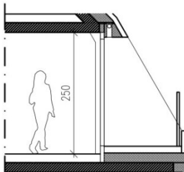
SCHNITT B
