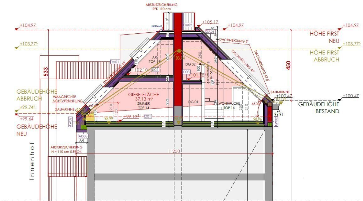
TEILSCHNITT D-D | M 1:100
