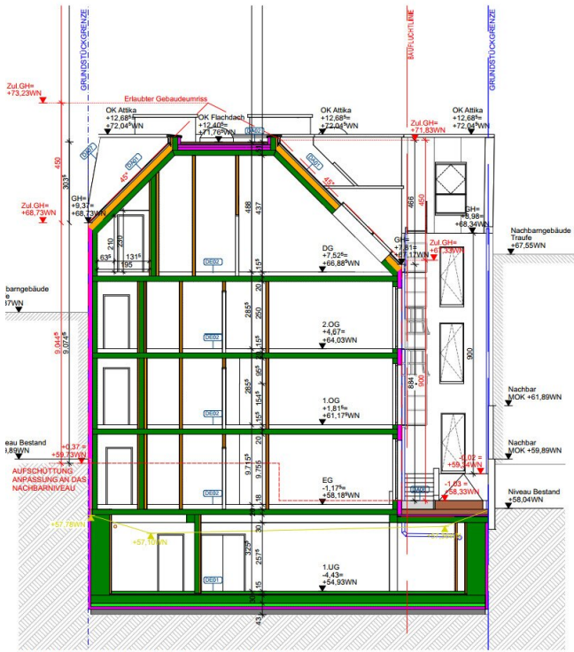
SCHNITT B-B 1:100
