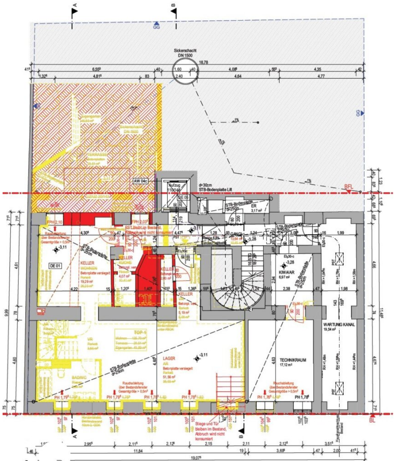
KELLERGESCHOSS
