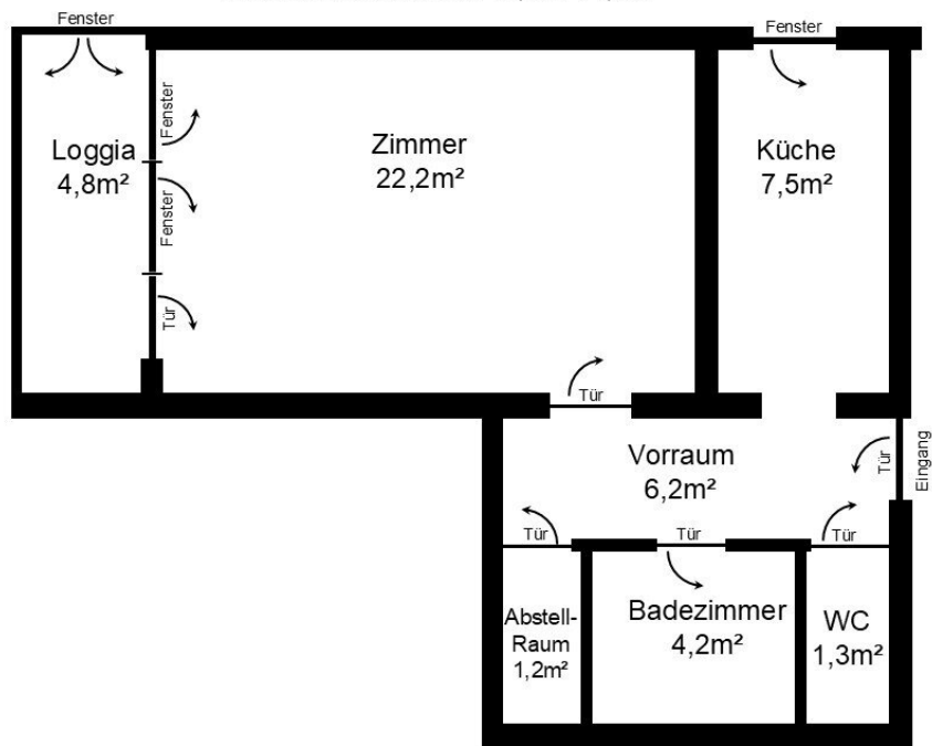
Skizze Grundriss ca.42,6m 2 +4,8m 2
