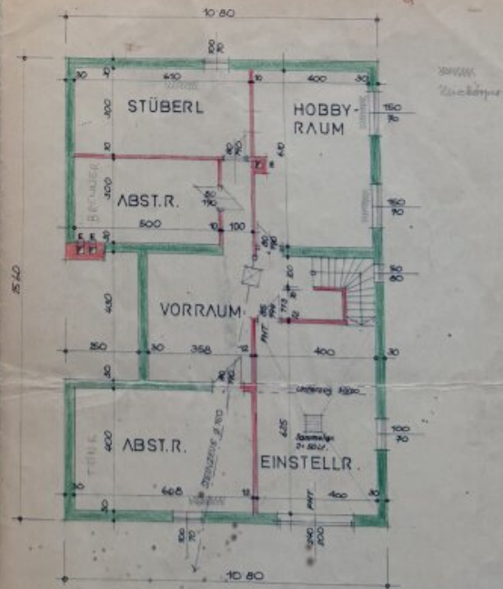
KELLERGEHOSS 1:100
