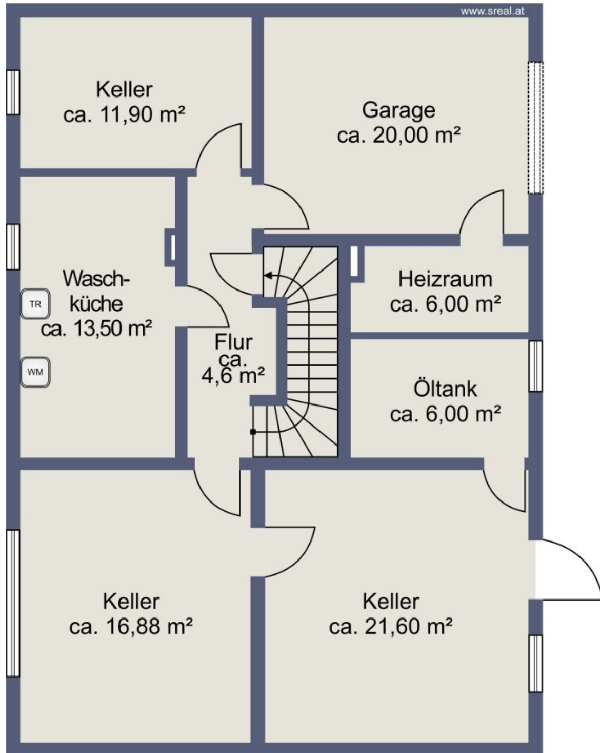
Planskizze Kellergeschoss
