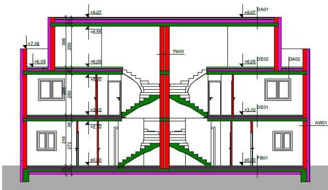
SCHNITT C-C
