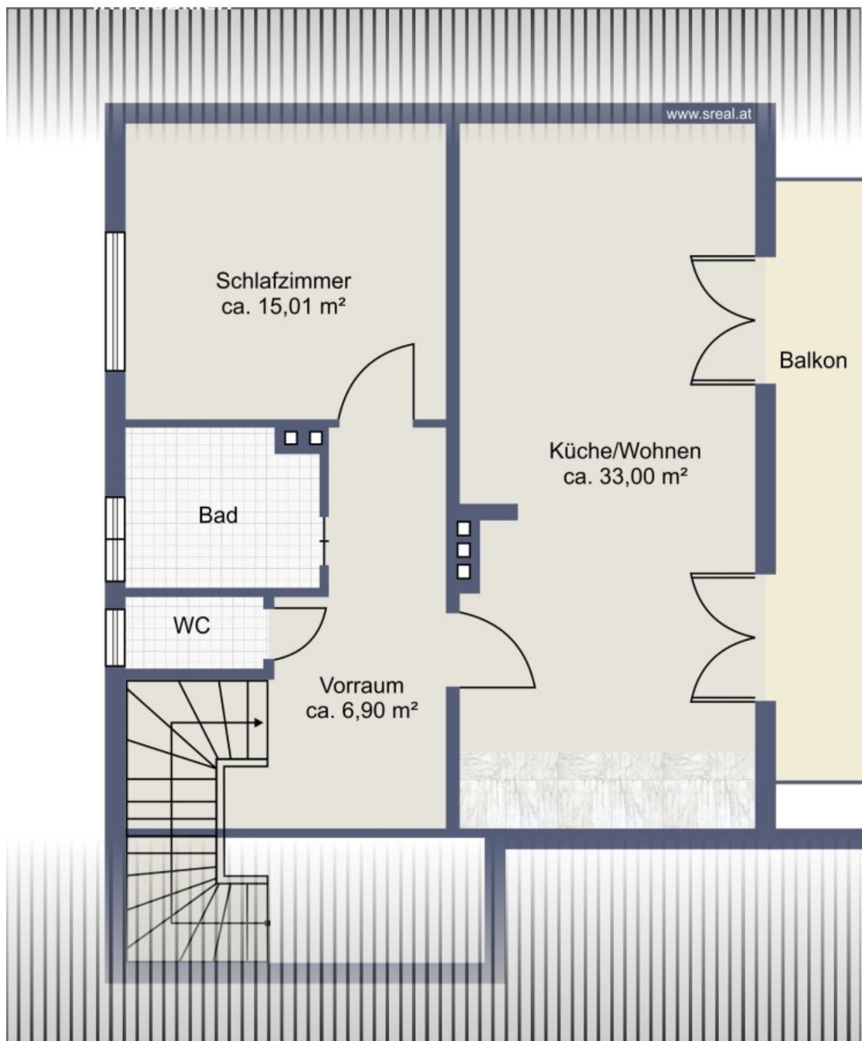
Skizze Dachgeschoss
