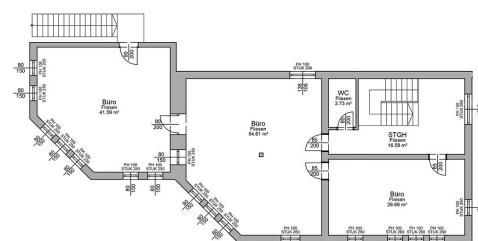
Grundriss Obergeschoss
