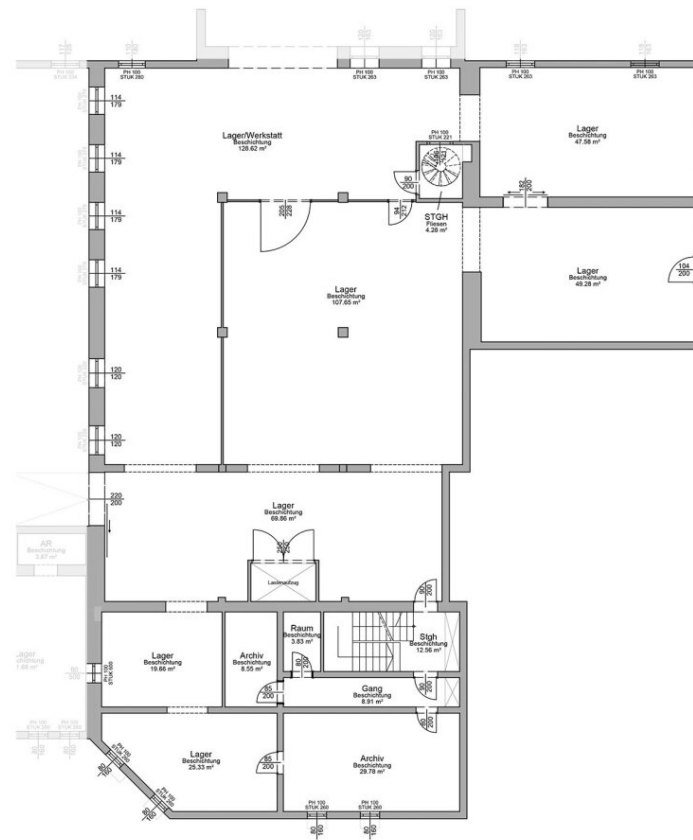
Grundriss Untergeschoss
