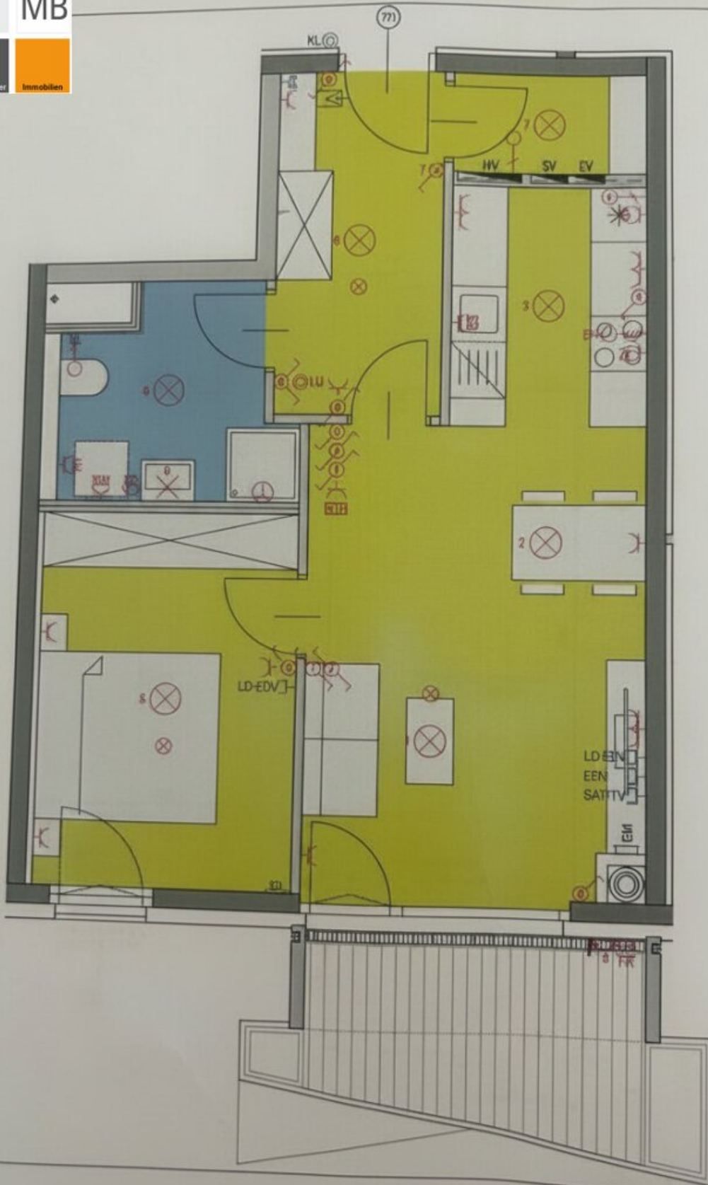
VERGABEPLAN TOP 721 I 3. OBERGESCHOSS
