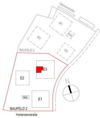
ÜBERSICHTSPLAN
