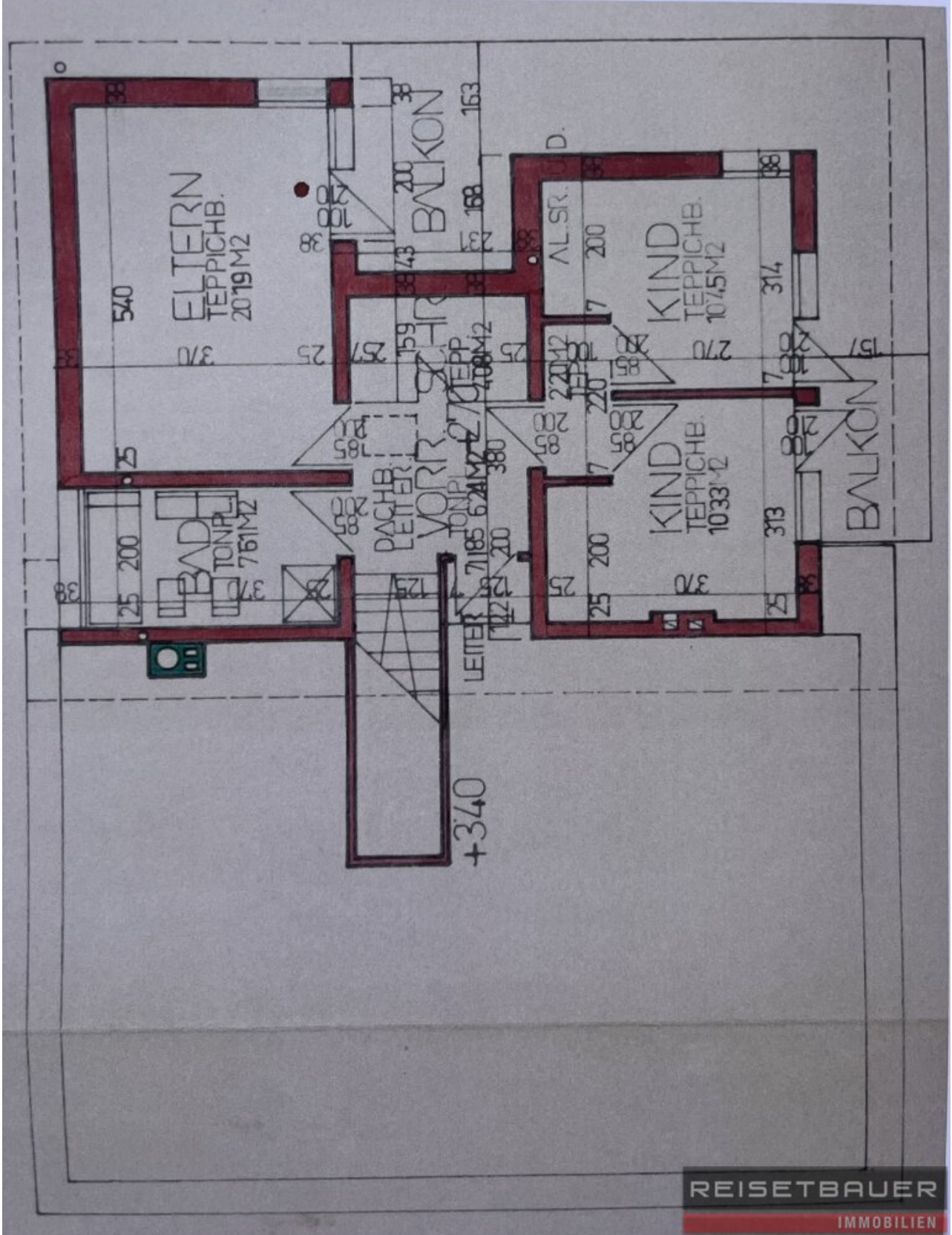
Grundrissplan Obergeschoss
