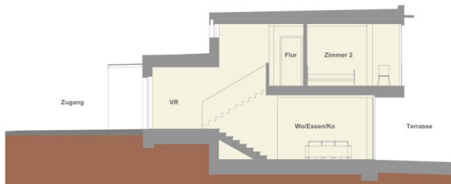
SCHNITT
