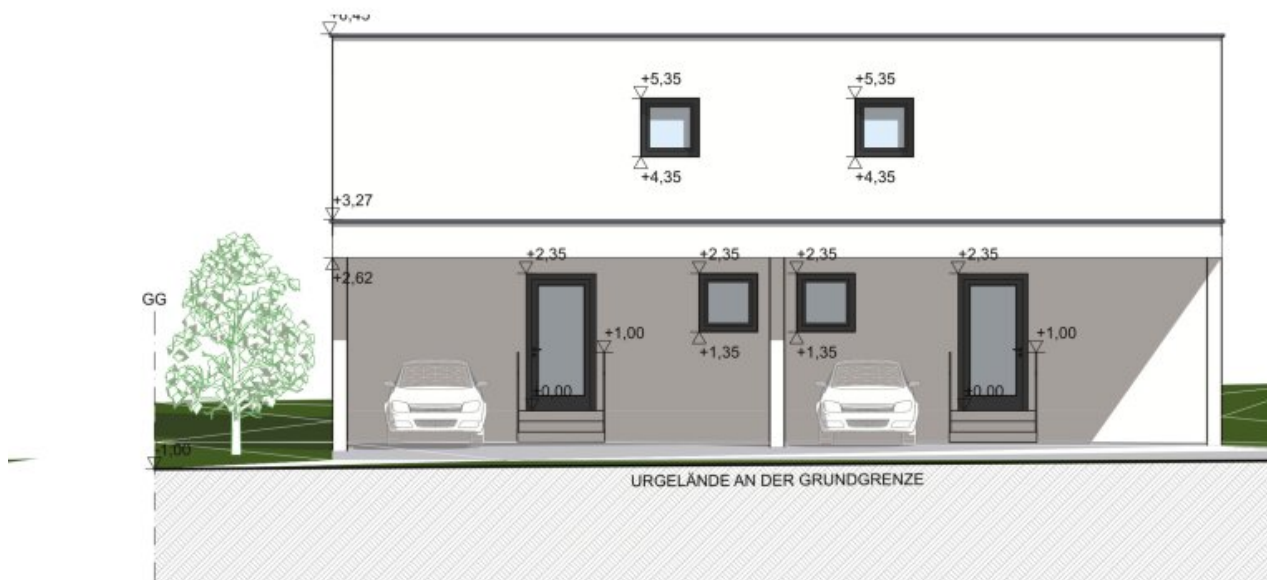
NW - Ansicht
