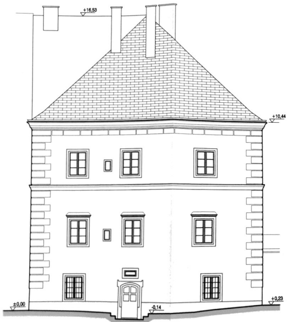
SÜDANSICHT
