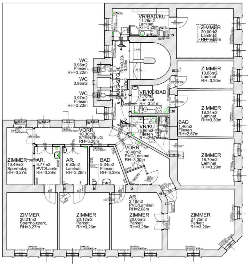
1. OBERGESCHOSS
