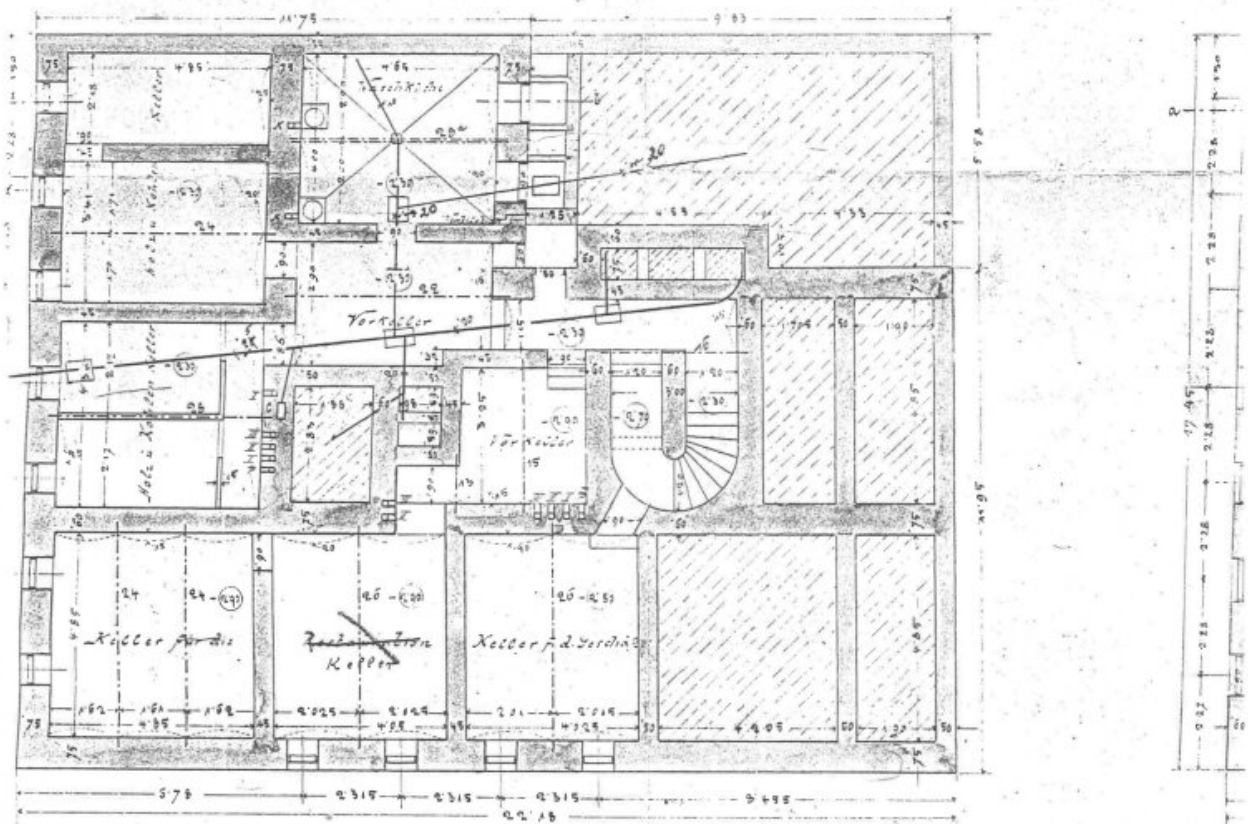
Keller & Fundament
