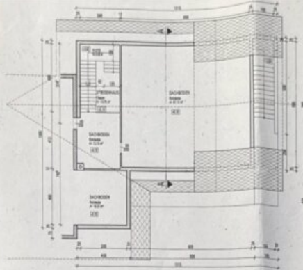
DACHGESCHOSS
