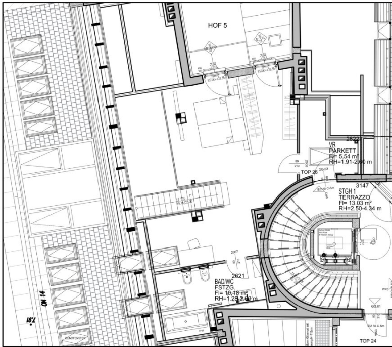
GALERIEGESCHOSS
