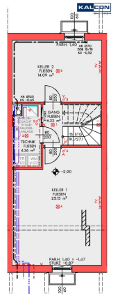
Kellergeschoss
