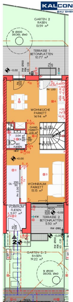
Erdgeschoss
