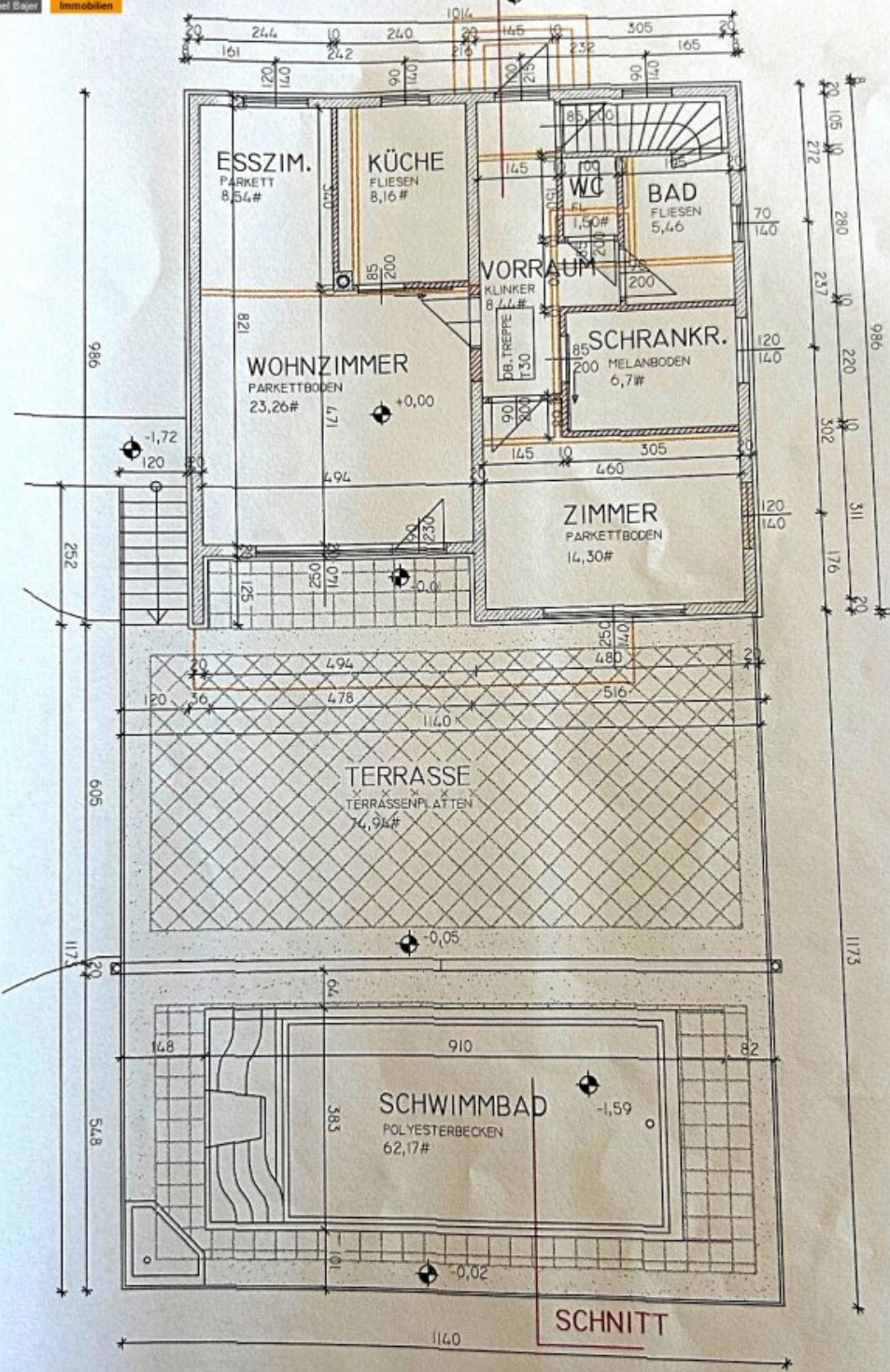
POLIERPLAN 1:50
