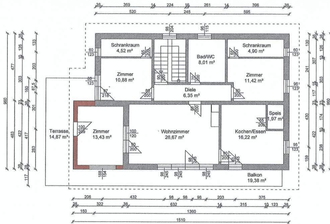
OBERGESCHOSS M=1/100
