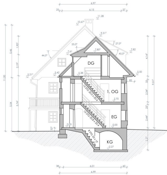
SCHNITT A-A
