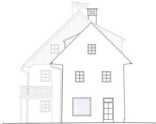
SÜDANSICHT
