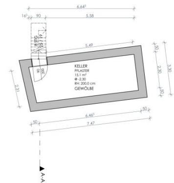
GRUNDRISS KG
