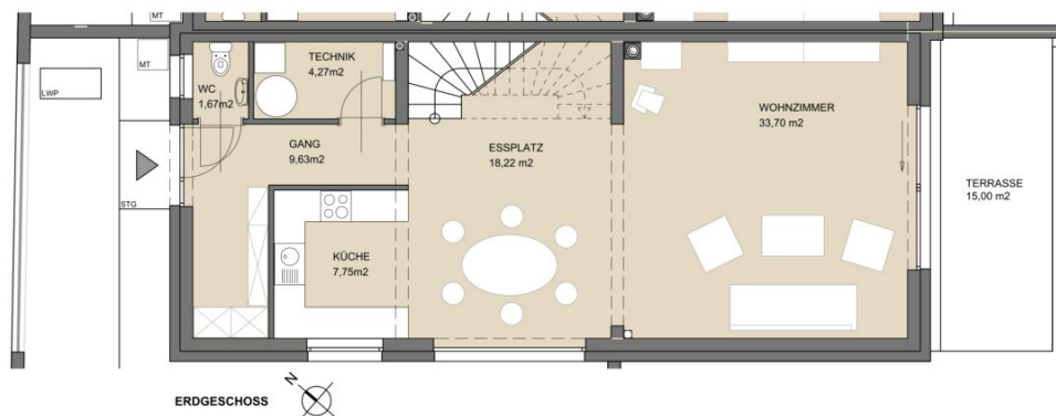
ERDGESCHOSS
