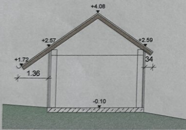
Nebengebäude Schnitt 1/1 M 1:100
