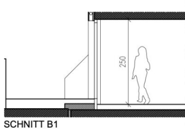
SCHNITT B1
