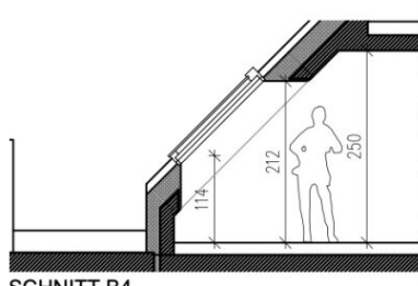
SCHNITT B4
