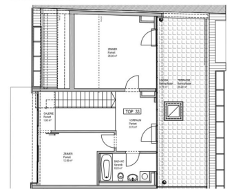
2. DACHGESCHOSS
