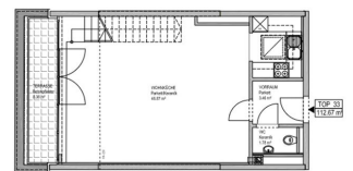
1. DACHGESCHOSS
