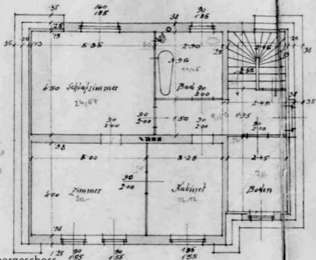
Obergeschoss
