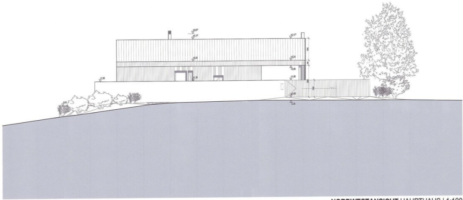
NORDWESTANSICHT HAUPTHAUS | 1:100
