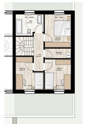
Obergeschoss 1/75
