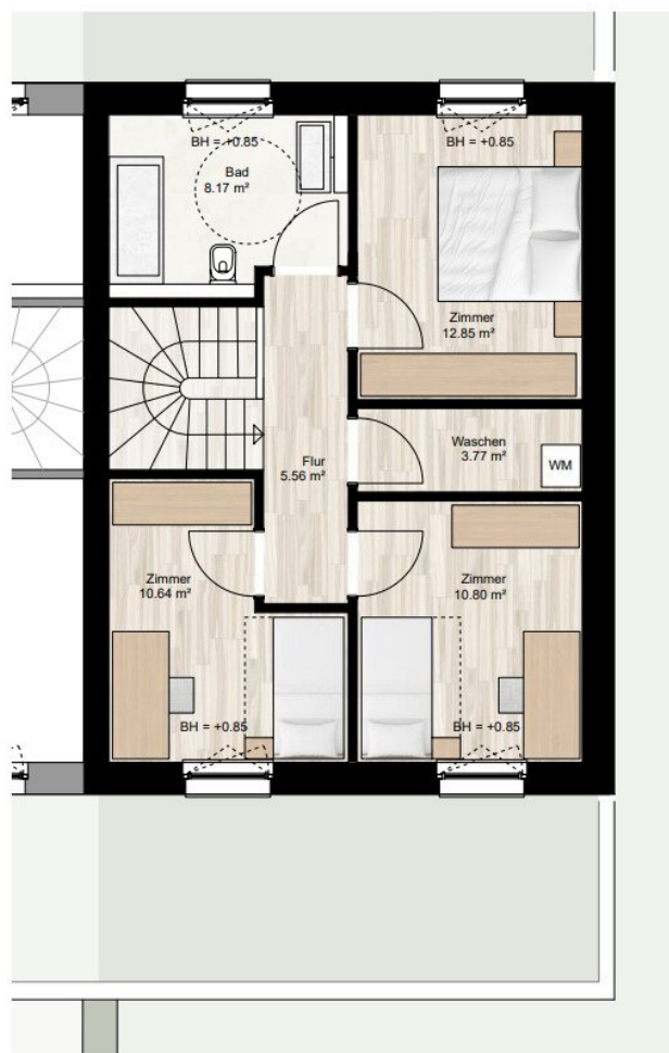
Obergeschoss 1/75
