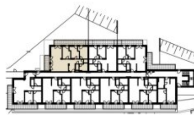
GRUNDRIS BK 03
